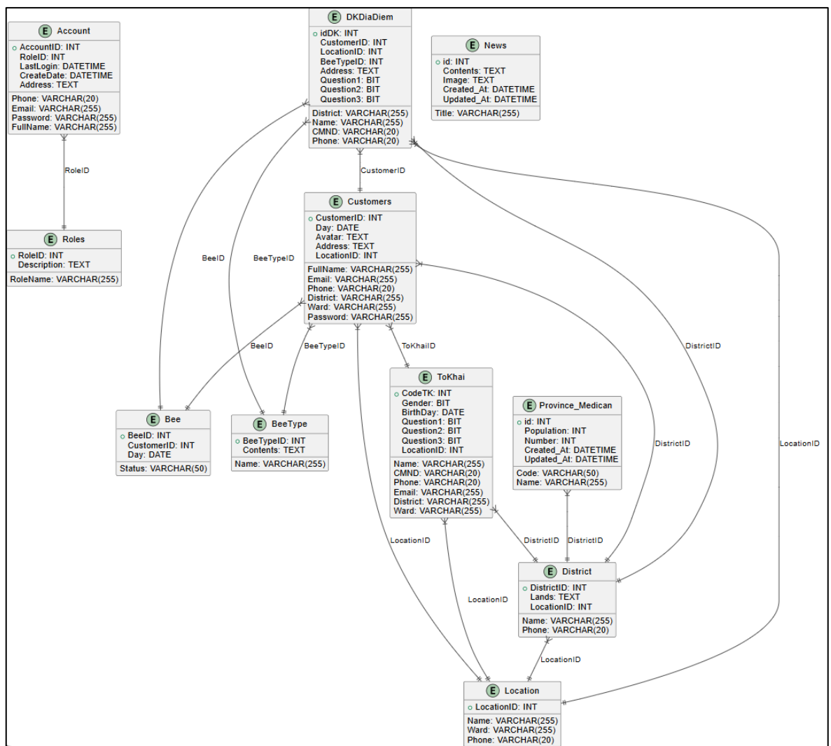
Hình 3. 8. Sơ đồ CSDL logic
