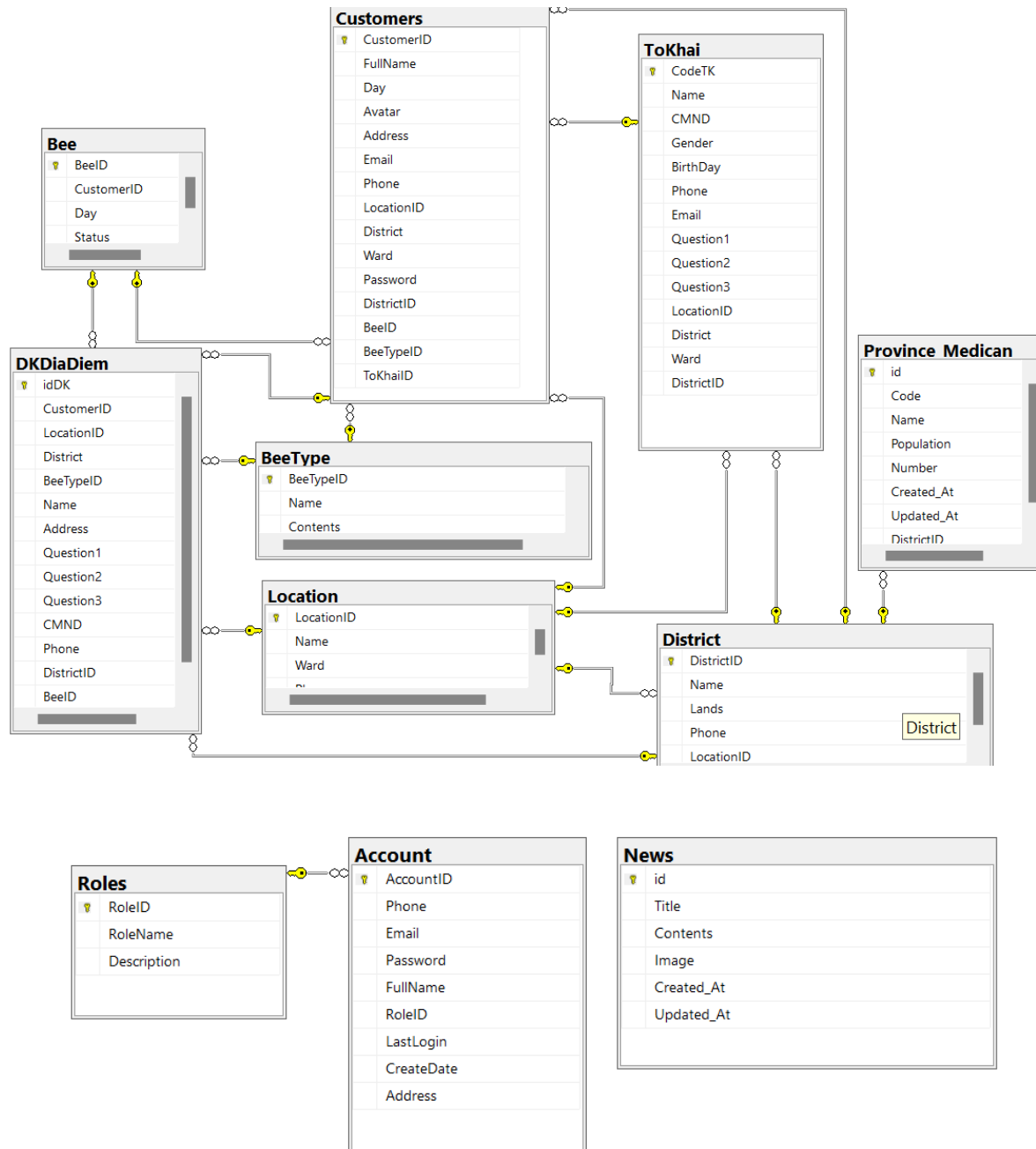
Hình 3. 7. Lược đồ CSDL quan hệ của truy vết các địa điểm đặt ong mật
