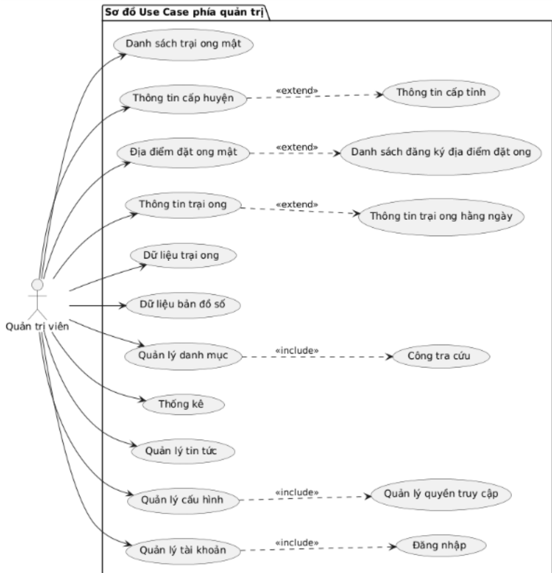
Hình 3. 4. Sơ đồ Use Case phía quản trị
