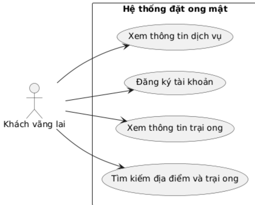
Hình 3. 6. Sơ đồ Use Case phía khách vẫn lại
