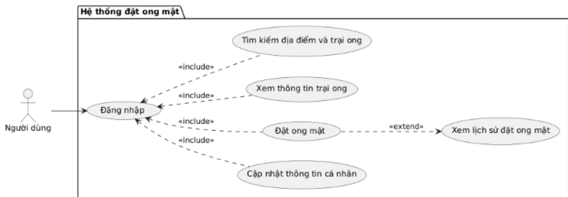
Hình 3. 5. Sơ đồ Use Case phía khách
