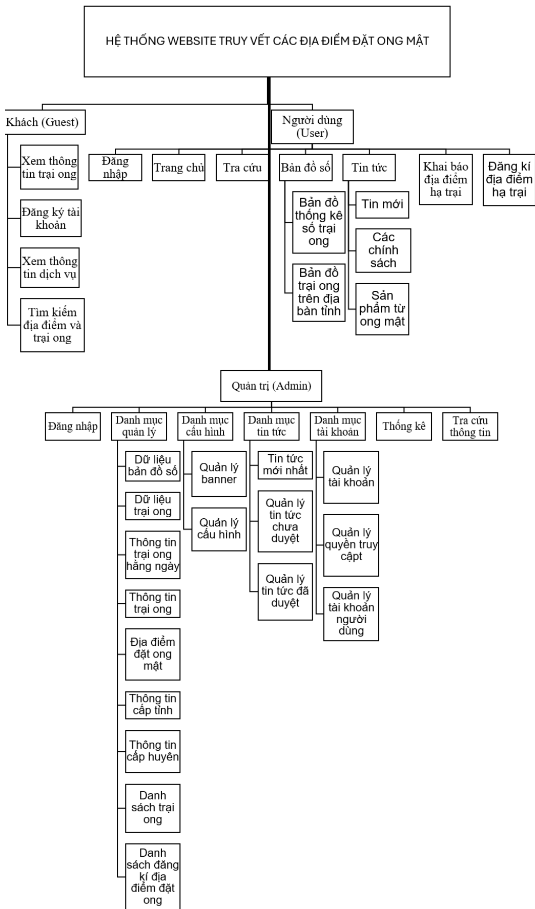
Hình 3. 1. Sơ đồ chức năng (Functional diagram)
