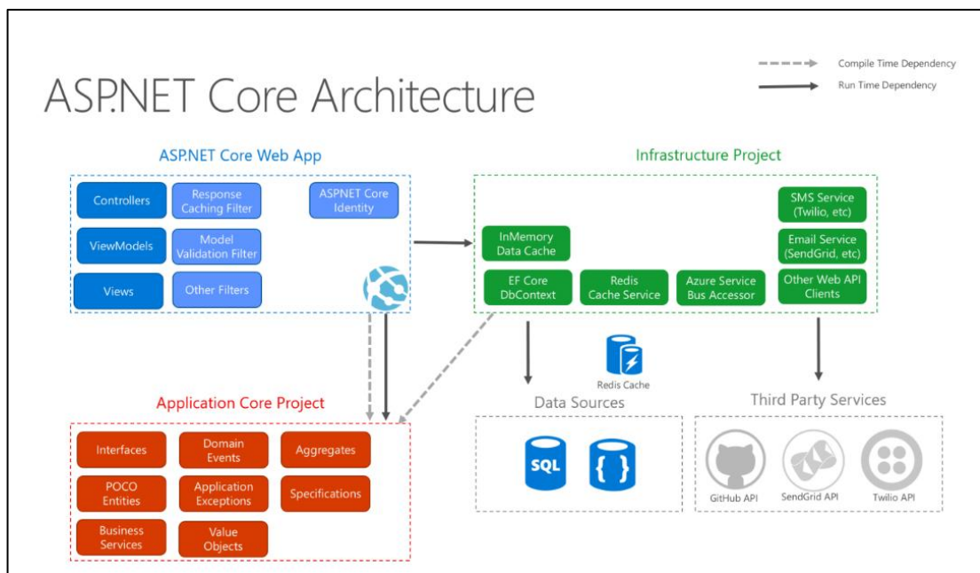
Hình 3. 2. Sơ đồ kiến trúc (Architecture diagram)
